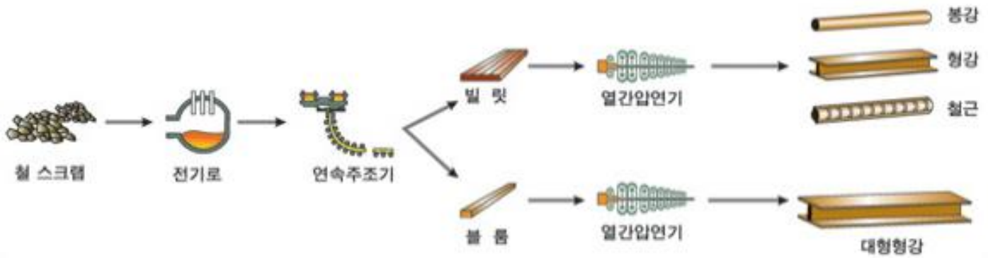
그림 5. 전기로 방식 제품 생산 과정
