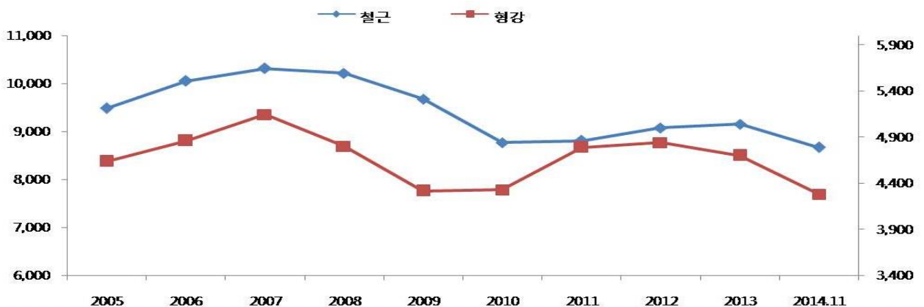
그림 7. 동사 철근 및 형강 생산량 추이
