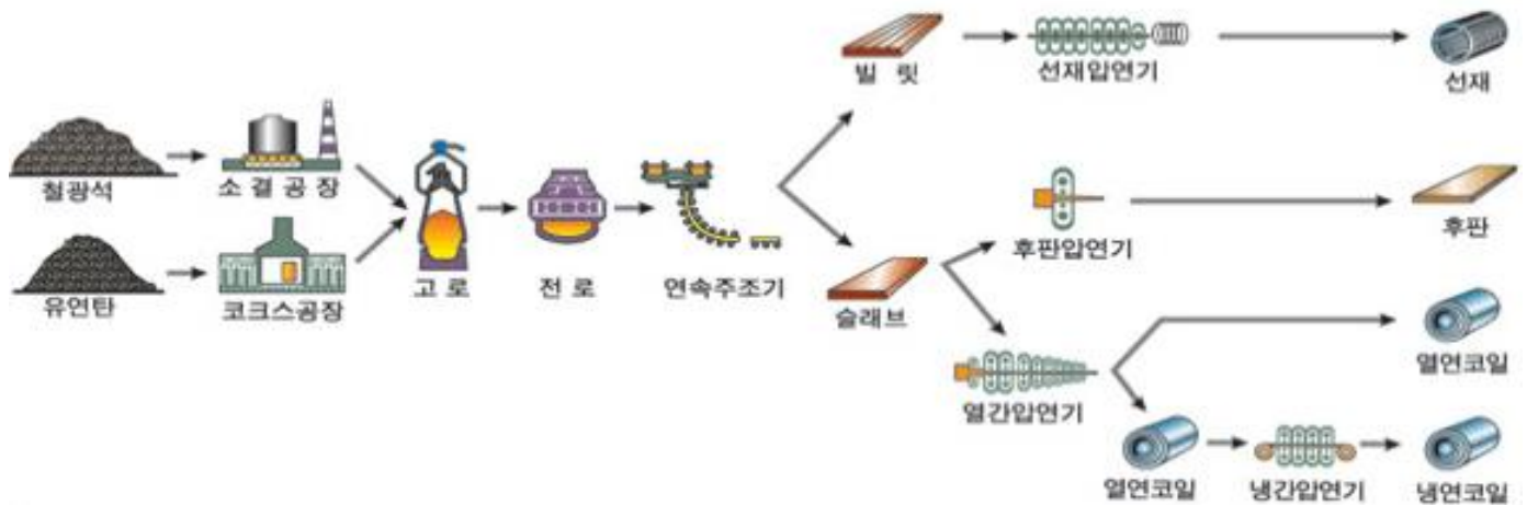
그림 4. 고로 방식 제품 생산 과정
