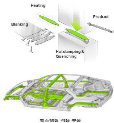
그림 19. 핫스탬핑 공법 및 적용분야
